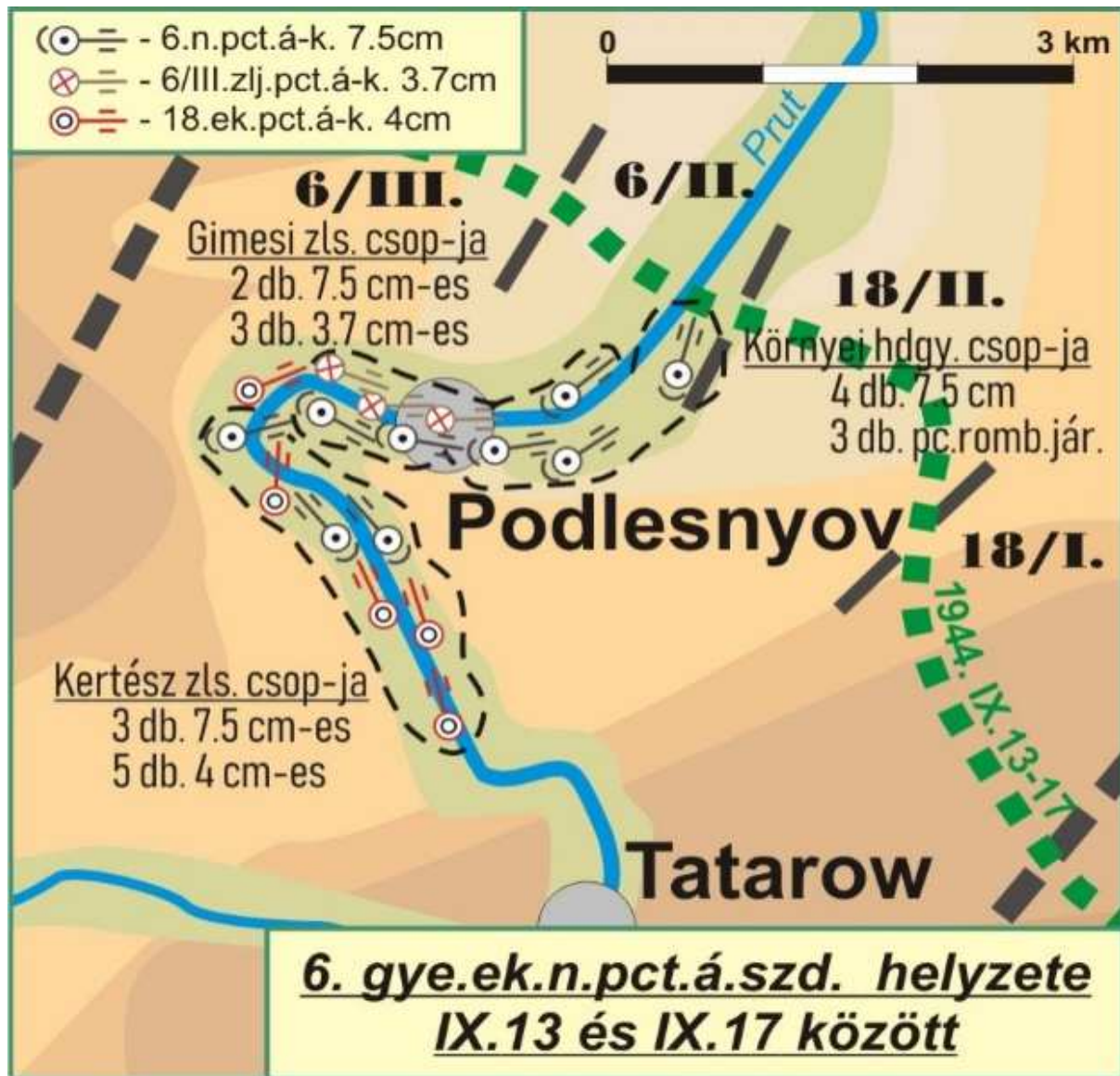
5. ábra. A 6. gyalogezred ezredközvetlen nehéz páncéltörő ágyús század helyzete 1944. szeptember 13–17. között 187
